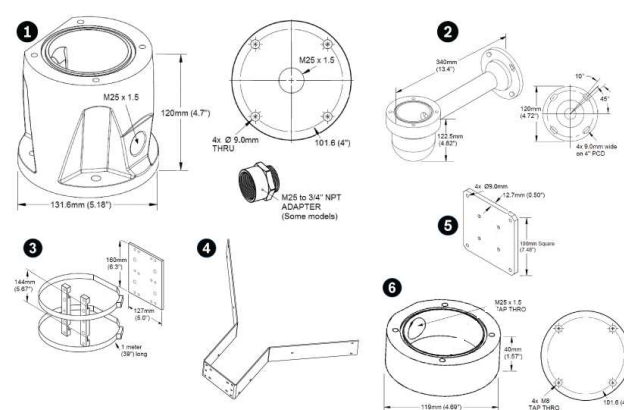
Fig. 1: Montages en option, série MIC IP 7100i
